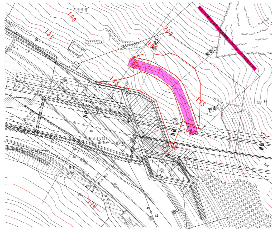
平面図 S=1:200
