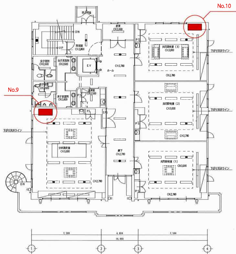
産業技術共同研究センター 3階 ドラフト配置図
