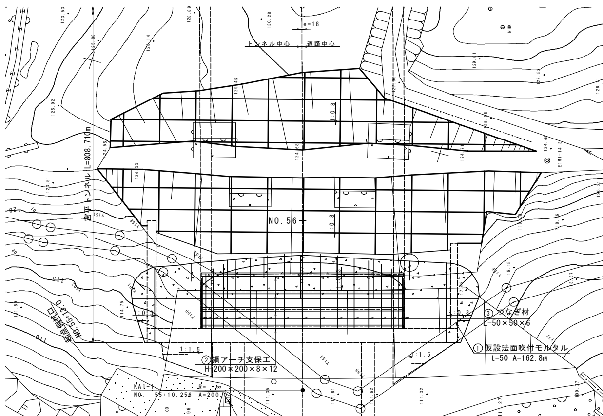
坑口付け工平面図
